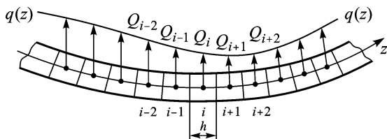
Рис. 2. Конечно-элементное представление участка трубопровода
